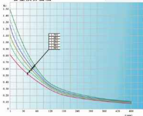
容量换算曲线
